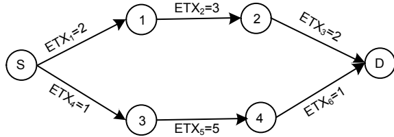
Fig. 3 ETX example
